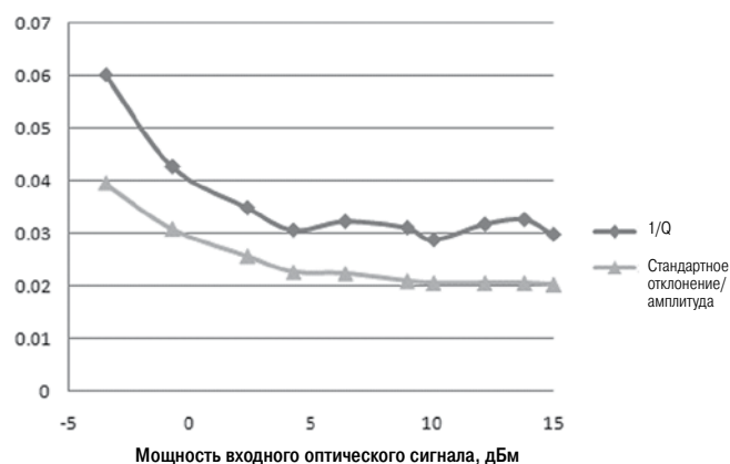
Рис. 19. Погрешность констелляционной диаграммы, включая погрешность интрадина и демодуляции, можно получить, разделив среднеквадратическую погрешность точек констелляции на амплитуду электрического поля для каждого поляризованного сигнала. Приведенные данные получены на передатчике 2,5 Гбод NRZ 1-pol QPSK с помощью дискретизатора Tektronix 1 MS072004.
