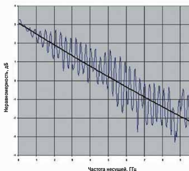
AWG7122C в режиме чередования Частота дискретизации 24 Гвыб./с
