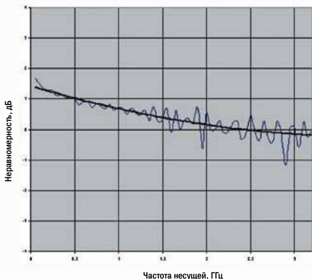
AWG7082C в стандартном/широкополосном исполнении Частота дискретизации 8 Гвыб./с
