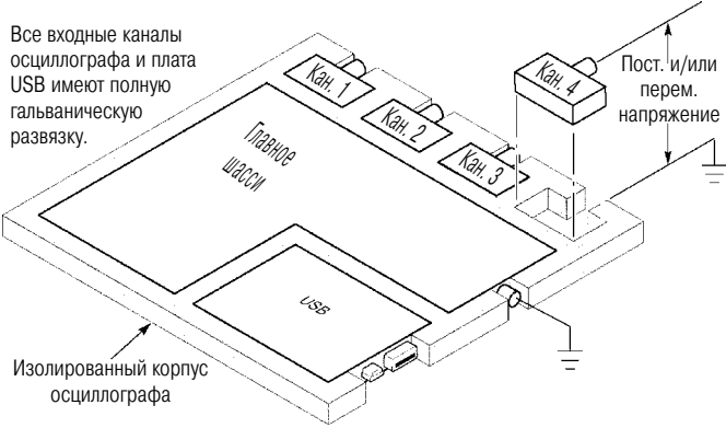
Максимальное напряжение относительно земли для входных каналов составляет 1000 В ср.кв. *
