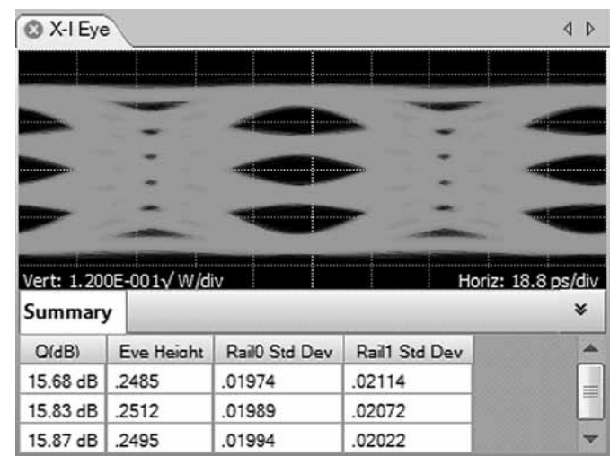
Рис. 12. Глазковая диаграмма поля.
