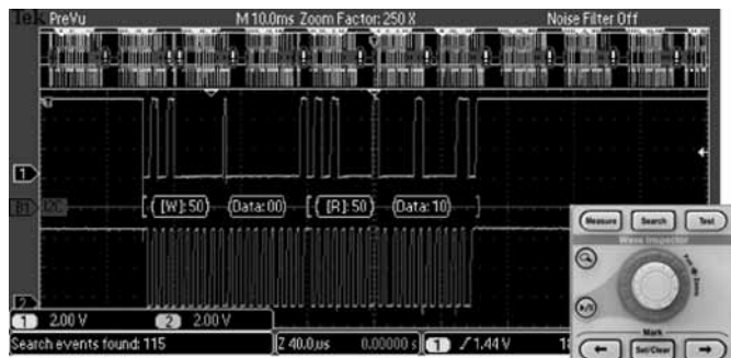
Поиск — Декодирование данных шины I 2 C с отображением результатов поиска адреса 50. Панель управления Wave Inspector обеспечивает непревзойденную эффективность при навигации и просмотре данных.
