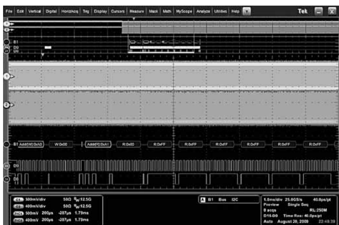
Захват длительностью 10 мс участков синхронных высокоскоростного и низкоскоростного сигналов с частотой дискретизации 25 Гвыб/с.
