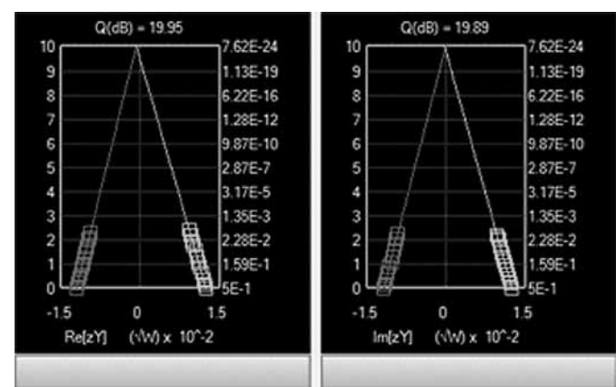
Рис. 7. Q-график.
