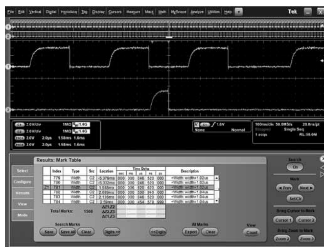
Шаг поиска 2. Wave Inspector осуществляет автоматический поиск по записи и отмечает каждое событие маркером в виде треугольника. После этого при помощи кнопок Previous (назад) и Next (вперед) можно перемещаться от одного события к другому.
