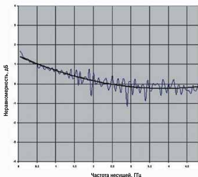
AWG7122C в стандартном/широкополосном исполнении Частота дискретизации 12 Гвыб./с
