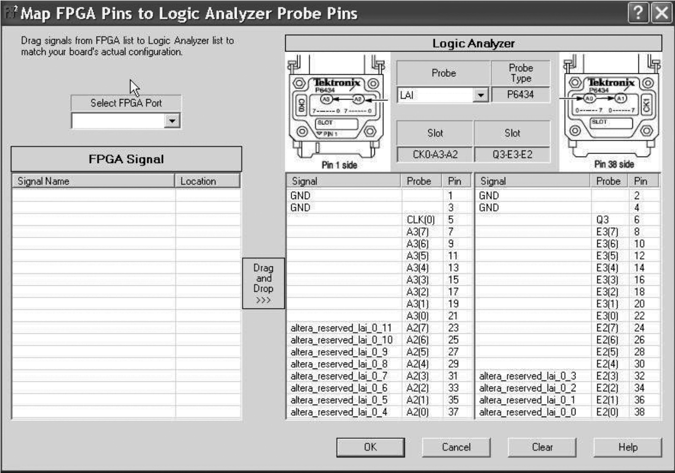
Рис. 6. FPGAView распределяет выводы быстро и просто.
