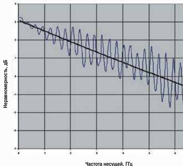
AWG7082C в режиме чередования Частота дискретизации 16 Гвыб./с
