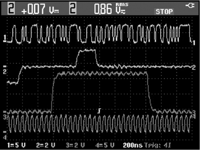
На экране осциллографа можно легко наблюдать любые смешанные сигналы, поступающие на 4 входных канала с полной гальванической развязкой.
