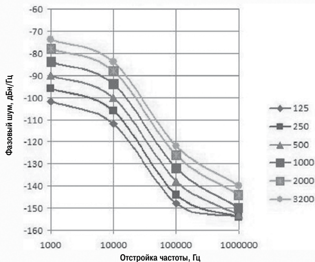
Фазовый шум (тип.) AWG7082C в стандартном и широкополосном исполнении.
