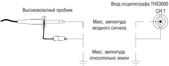
Максимальные значения входного сигнала и потенциала относительно земли.
