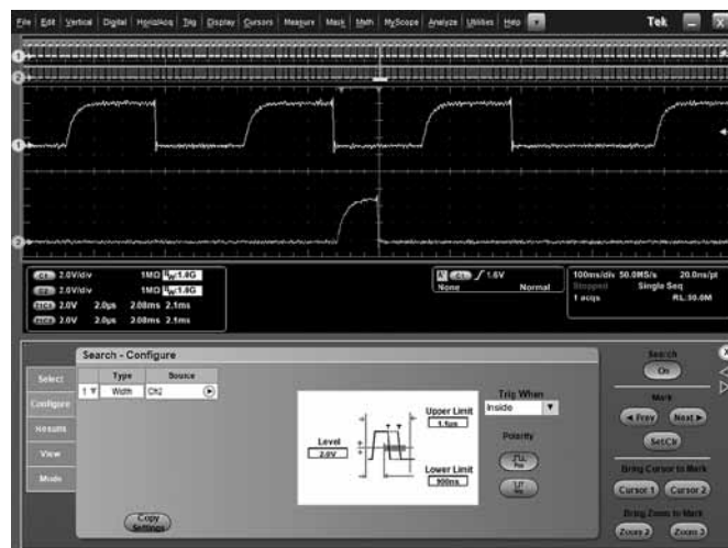
Шаг поиска 1. Определяем критерии поиска.
