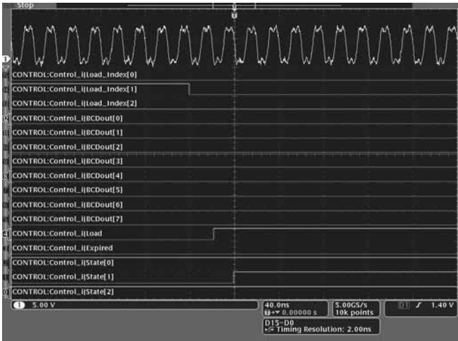
Рис. 8а. Осциллограф смешанных сигналов серии MSO4000 и ПО FPGAVIEW упрощают отладку ПЛИС.
