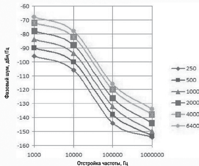
Фазовый шум (тип.) AWG7082C в режиме чередования.
