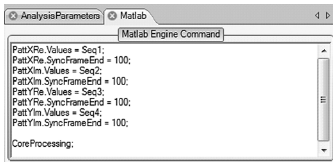
Рис 14. Окно MATLAB.
