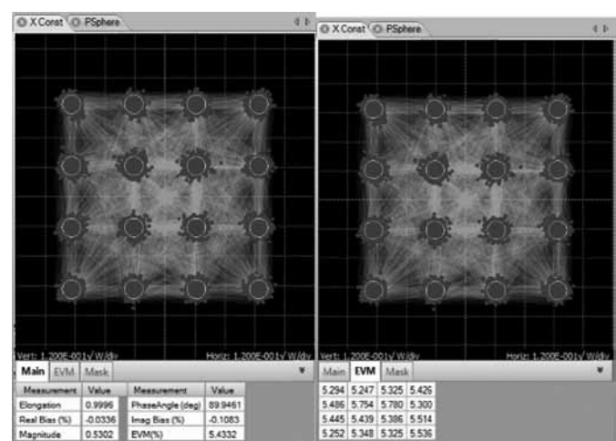
Рис. 8. Констанционная диаграмма.
