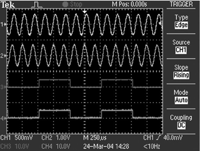
Четыре входа, выполненные по технологии IsolatedChannel™, и вход внешнего запуска позволяют быстро и точно выполнять измерения с гальванической развязкой от земли и измерения дифференциальных сигналов.
