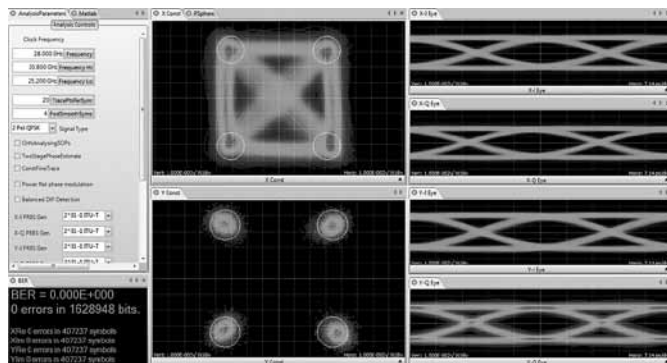
Рис. 1. Интерфейс пользователя (OUI) анализатора OM4000 отображает некоторые параметры градиациями цвета. Можно также применить цветовое кодирование символов в зависимости от предыдущего состояния. Показаны данные сигнала 112 Гбит/с PM-QPSK.
